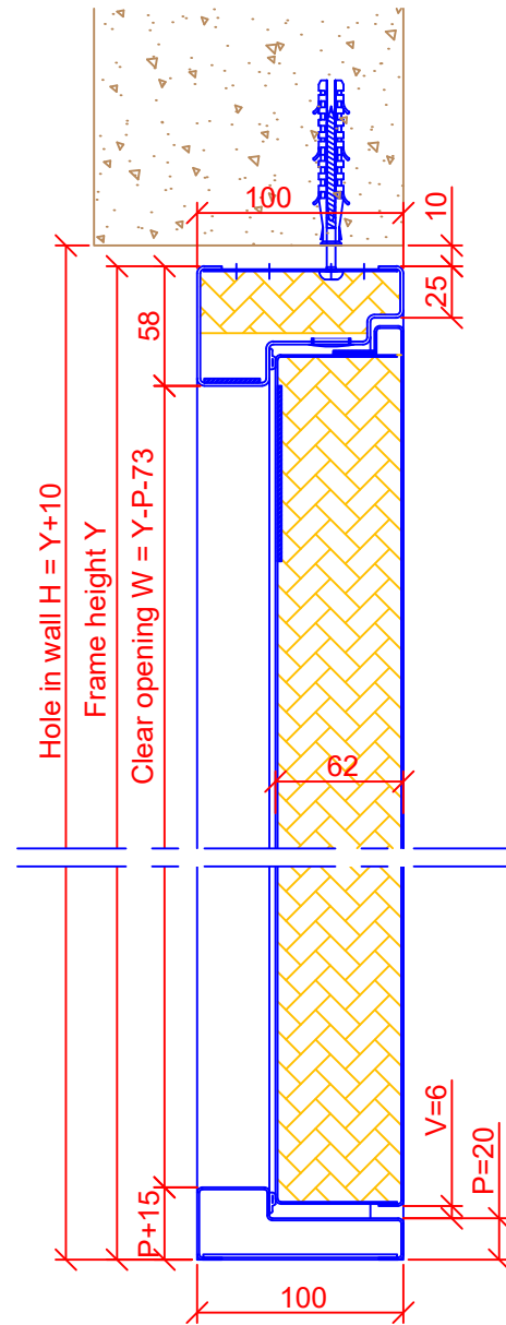
Sill P20/35 Section B-B (1 : 4)
